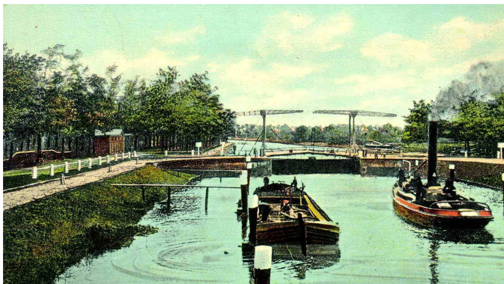
Naar binnen schuttend een modderbak, geassisteerd door een stoomsleeptboot, in de grote kolk van de Katerveersluizen, 1908.
