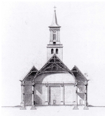
Apeldoorn, project A voor een simultaankerk van F.L. Gunckel uit 1810. Links: Opstand voorgevel. Rechts: Doorsnede door de breedte.
