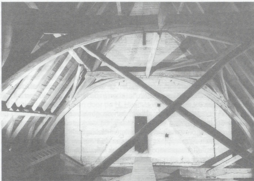
Oostzijde toren met dakmoet van het vorige schip en op de voorgrond de kap van het huidige schip. Foto archief RDMZ, A.J. van der Wal, mei 1994
