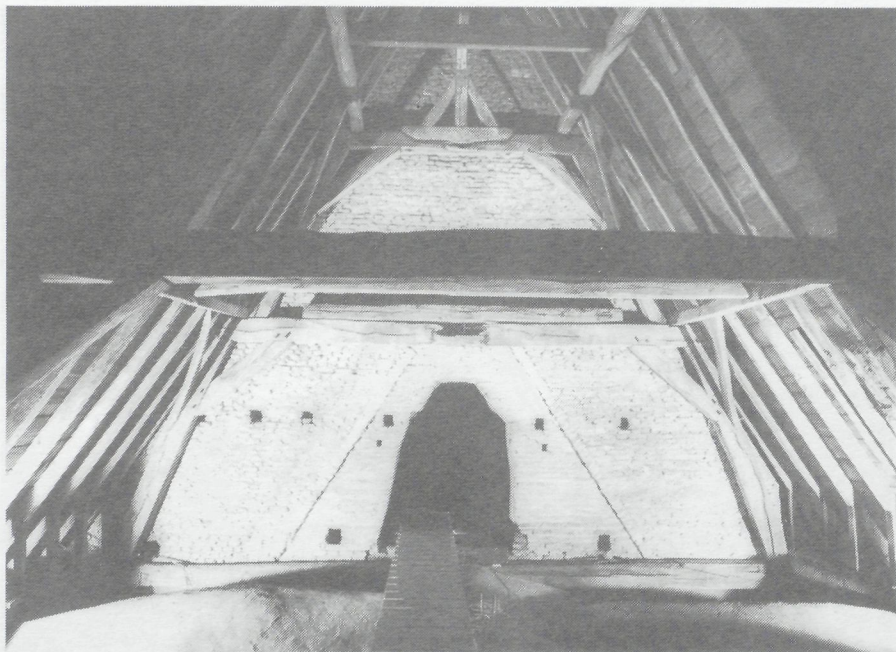
Oostzijde van de muur tussen koor en schip. In het midden is de dakmoet van het vorige schip zichtbaar. Foto archief RDMZ, A.J. van der Wal, mei 1994
